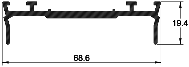
90-221 AĞIRLIK : 0.673 kg/mt.
