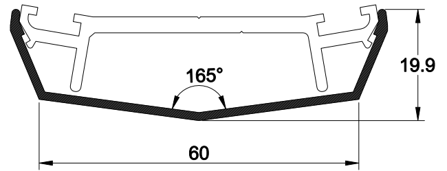
94-651 AĞIRLIK : 0.388 kg/mt.
