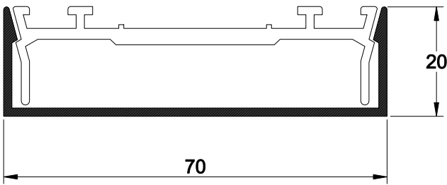
91-369 AĞIRLIK : 0.441 kg/mt.
