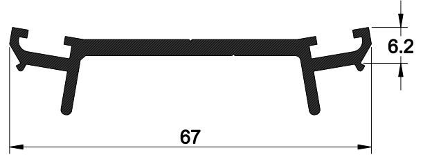
94-650 AĞIRLIK : 0.675 kg/mt.
