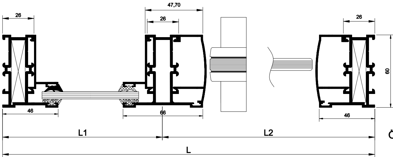
A-A Kesiti
