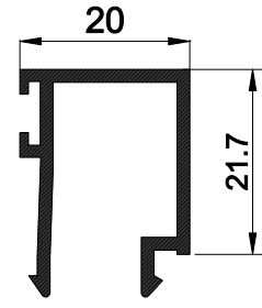
40 E 75 AĞIRLIK : 0.323 kg/mt.
