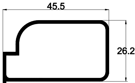
40 E 85 AĞIRLIK : 0.502 kg/mt. JX: 19.67 cm 4 JY: 46.59 cm 4
