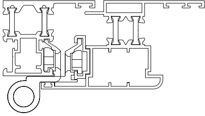
40 D 22 MENTEŞE Ö:1/2
