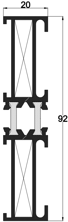
40 E 10 AĞIRLIK : 1.248 kg/mt. JX: 33.56 cm 4 JY: 1.49 cm 4
