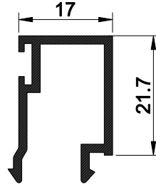
40 E 74 AĞIRLIK : 0.313 kg/mt.
