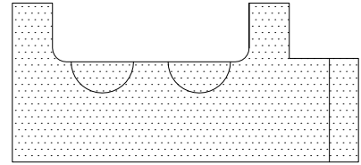
40 D 02 (3mm için) E.P.D.M. DIŞ CAM FİTİLİ
