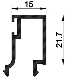
40 E 73 AĞIRLIK : 0.310 kg/mt.
