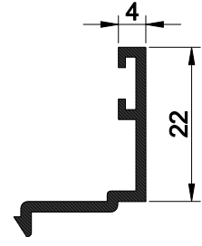
40 E 71 AĞIRLIK : 0.197 kg/mt.
