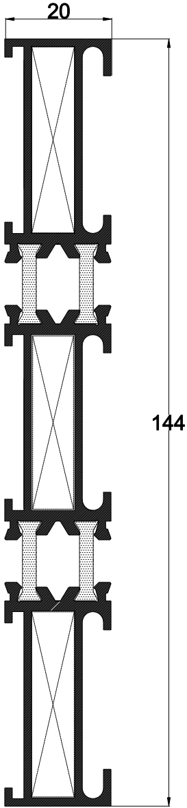
40 E 11 AĞIRLIK : 2.000 kg/mt. JX: 118.77 cm 4 JY: 2.33 cm 4
