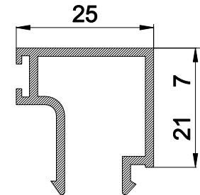
40 E 78 AĞIRLIK : 0.359 kg/mt.
