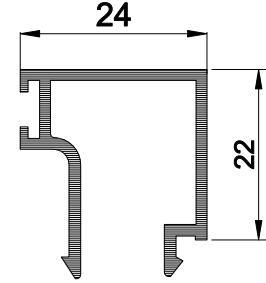
40 E 72 AĞIRLIK : 0.340 kg/mt.
