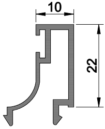
40 E 70 AĞIRLIK : 0.275 kg/mt.
