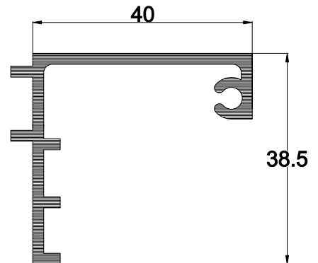
40 E 62 AĞIRLIK : 0.610 kg/mt.
