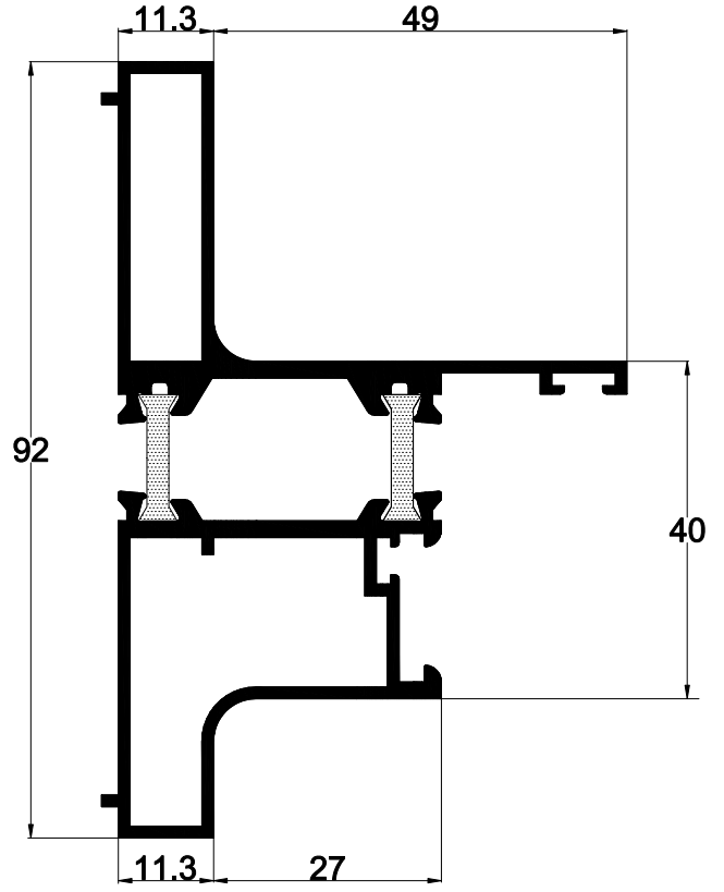
40 E 50 AĞIRLIK : 1.624 kg/mt. JX: 29.43 cm 4 JY: 13.48 cm 4
