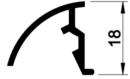
40 E 86 AĞIRLIK : 0.180 kg/mt.
