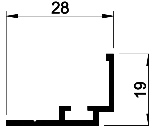
40 E 87 AĞIRLIK : 0.195 kg/mt.
