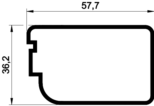
50 E 87 AĞIRLIK : 0.768 kg/mt. JX: 5.82 cm 4 JY: 12.15 cm 4
