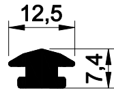
05-2306 AĞIRLIK : 0.160 kg/mt
