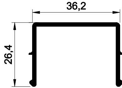
50 E 84 AĞIRLIK : 0.385 kg/mt.
