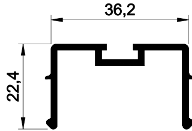
50 E 85 AĞIRLIK : 0.397 kg/mt.
