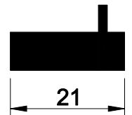
50 E 98 AĞIRLIK : 0.420 kg/mt.
