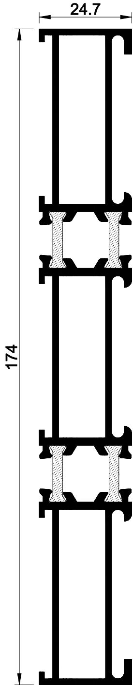
50 E 37 AĞIRLIK : 2.352 kg/mt. JX: 234.60 cm 4 JY: 5.18 cm 4
