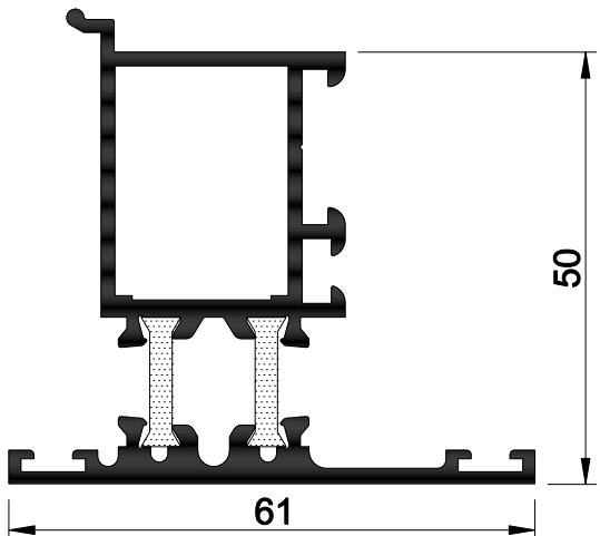
50 E 33 AĞIRLIK : 1.291 kg/mt. JX: 13.70 cm 4 JY: 7.53 cm 4
