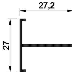
00-1322 AĞIRLIK : 0.185 kg/mt.
