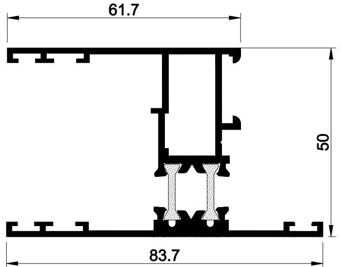
50 E 35 AĞIRLIK : 1.484 kg/mt. JX: 19.69 cm 4 JY: 18.47 cm 4
