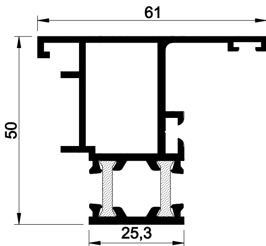
50 E 31 AĞIRLIK : 1.187 kg/mt. JX: 12.61 cm 4 JY: 7.30 cm 4
