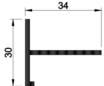
92-447 AĞIRLIK : 0.346 kg/mt.
