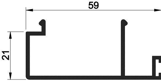
50 E 83 AĞIRLIK : 0.558 kg/mt.
