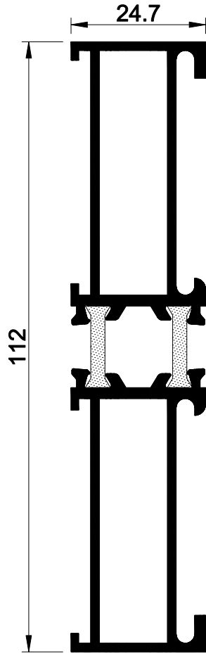
50 E 34 AĞIRLIK : 1.623 kg/mt. JX: 67.06 cm 4 JY: 3.33 cm 4
