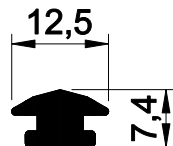
05-2306 Ağırlık: 0.160 kg/mt (Yüzey işlemsiz kullanılır)
