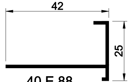
40 E 88 AĞIRLIK : 0.255 kg/mt.
