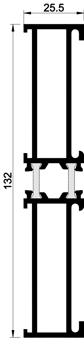
60 E 34 AĞIRLIK : 1.921 kg/mt. JX: 123.69 cm 4 JY: 4.42 cm 4
