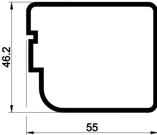
60 E 87 AĞIRLIK : 0.932 kg/mt. JX: 10.86 cm 4 JY: 14.36 cm 4
