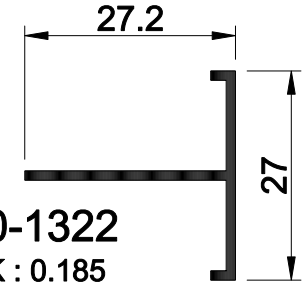
60 E 85 AĞIRLIK : 0.491 kg/mt.
