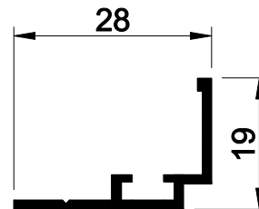
40 E 87 AĞIRLIK : 0.195 kg/mt.
