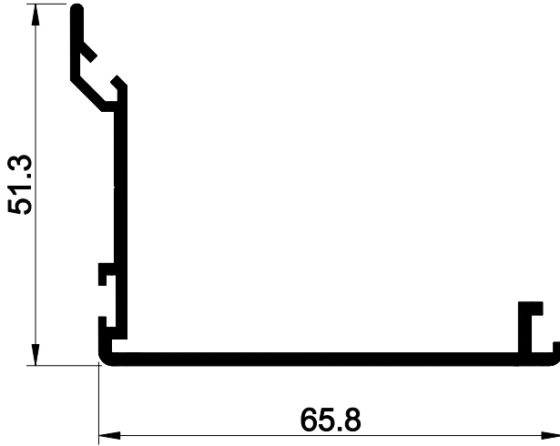
60 E 86 AĞIRLIK : 0.649 kg/mt.
