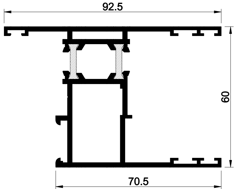
60 E 35 AĞIRLIK : 1.926 kg/mt. JX: 36.36 cm 4 JY: 28.20 cm 4
