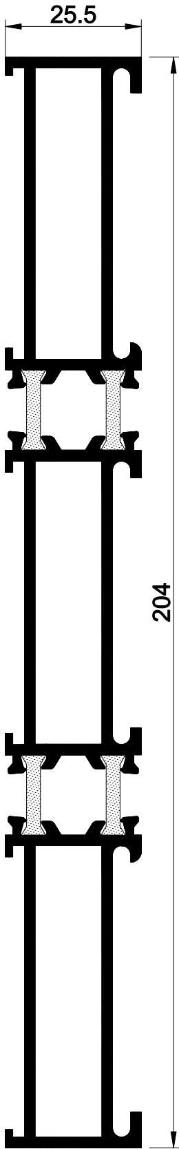
60 E 37 Ağırlık: 3.060 kg/mt JX: 422.94 cm 4 JY: 6.78 cm 4
