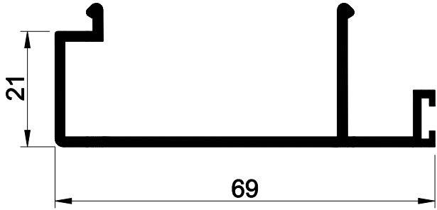
60 E 83 AĞIRLIK : 0.667 kg/mt.
