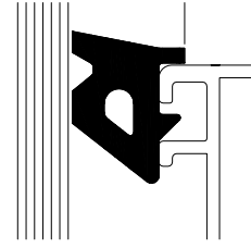
HY-4 İÇ CAM FİTİLİ (6+12+6 CAM KALINLIĞINA GÖRE) (SABİT KISIMLARDA)
