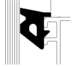
HY-4 İÇ CAM FİTİLİ (6+12+6 CAM KALINLIĞINA GÖRE) (SABİT KISIMLARDA)
